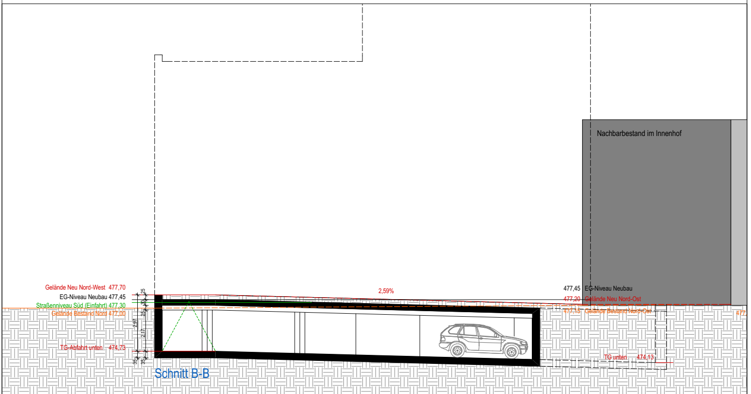
Schnitt B-B, 1-200
