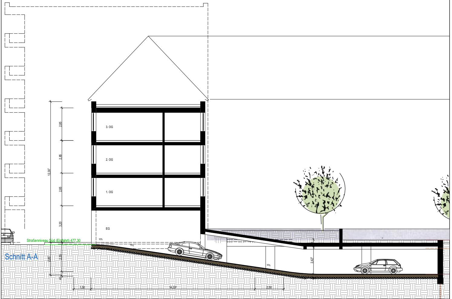
Schnitt A-A, 1-200
