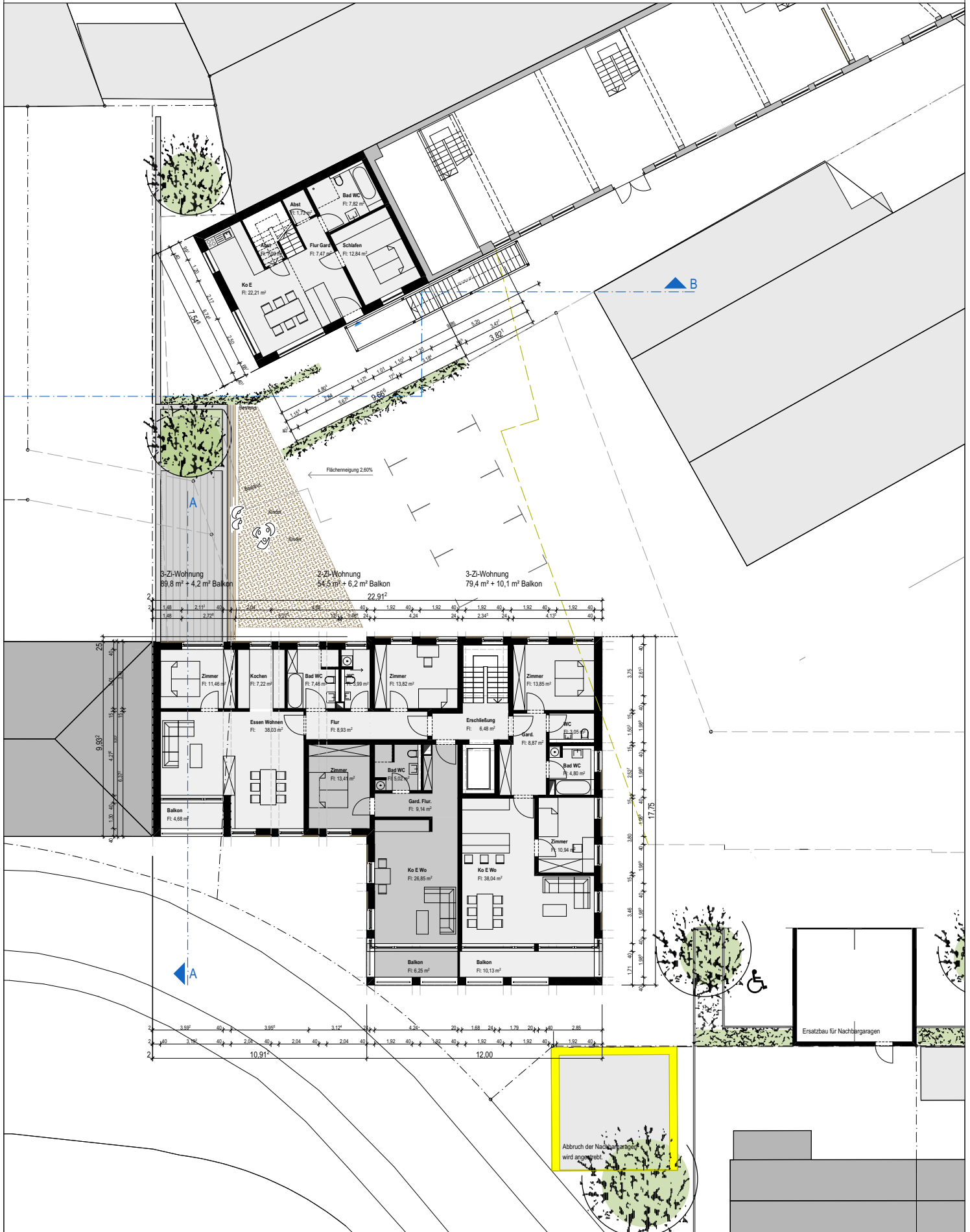
BA I Obergeschosse 1-3, BA II Obergeschoss 1, 1-250
